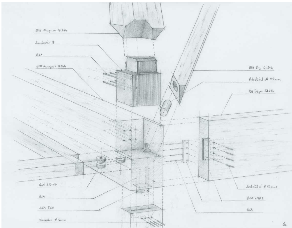
Abbildung 6: Auflagerknoten Skizze: Lukas Eschmann, Meili, Peter &amp; Partner Architekten AG, Zürich
