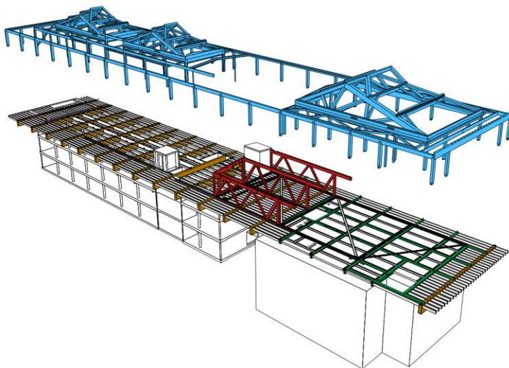
Abbildung 1: Konstruktion
