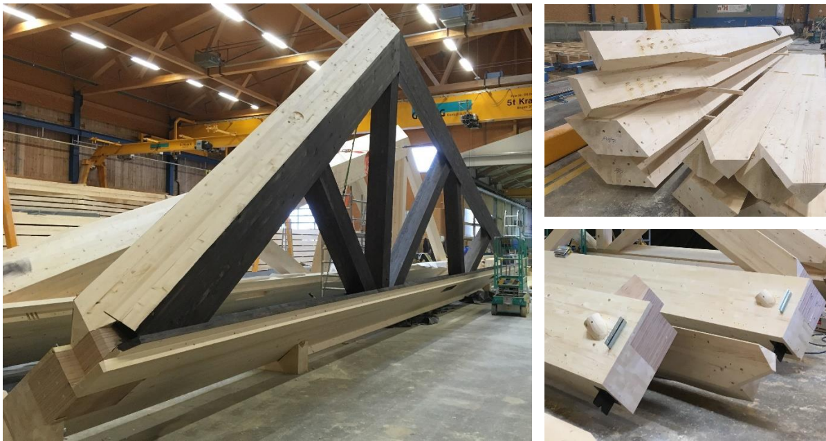
Abbildung 7: Fachwerkbauwerke Fotografie: neue Holzbau AG, Lungern
