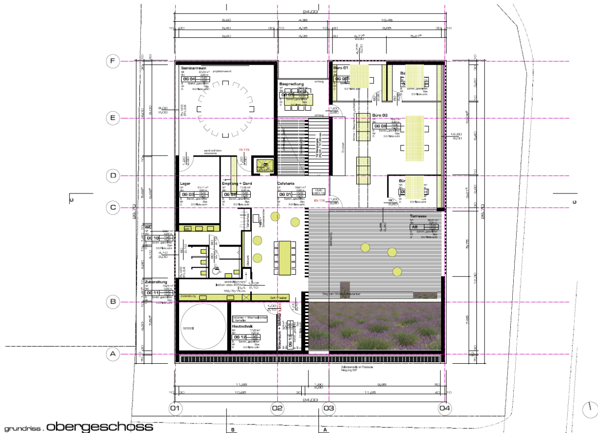
Abbildung 3: OG Grundriss Einreichung Aromacampus (Ventira Architekten)
